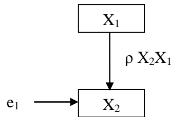
Gambar 3.2 Diagram Analisis Jalur Sub-Struktur 1
