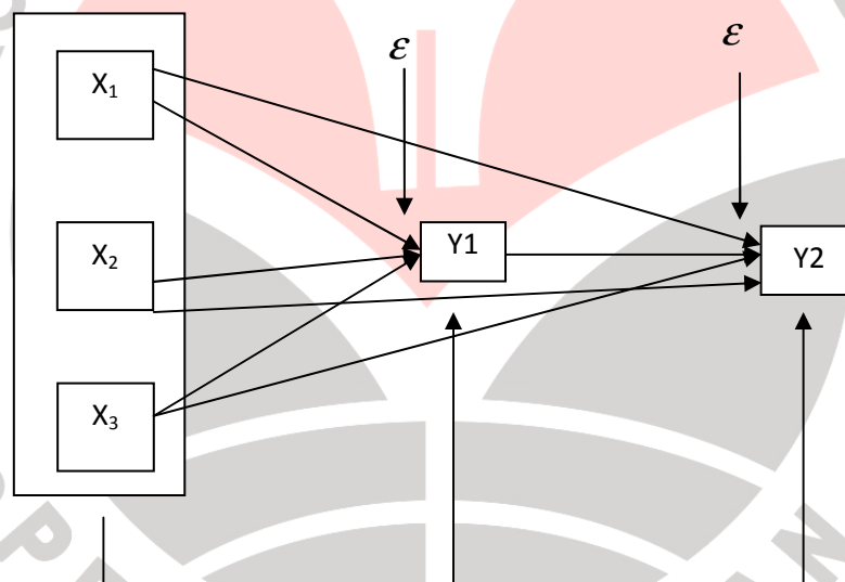
Gambar 3.2 Struktur Kausal Antara X_1 , X_2 , X_3 , Y_1 dan Y_2
