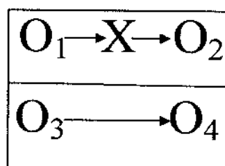
Gambar 3.1 Skema Penelitian
