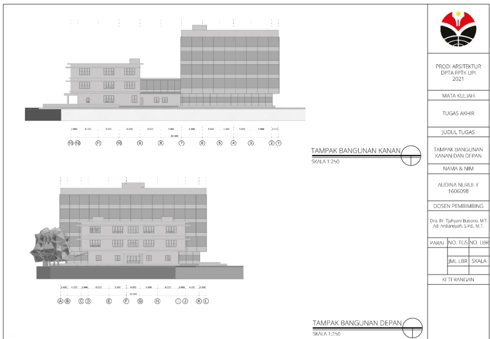
Gambar 5. 12 Tampak Bangunan Kanan dan Depan
