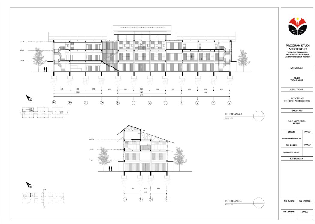
Gambar 5.13 Potongan Gedung Administrasi
