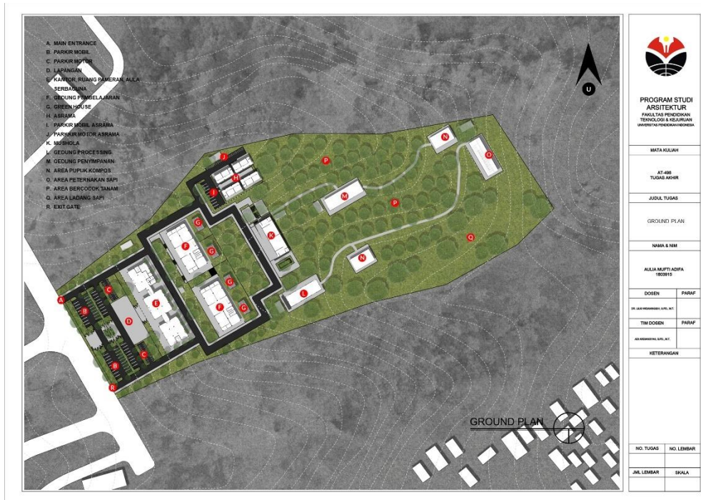
Gambar 5.1 Rencana Tapak
