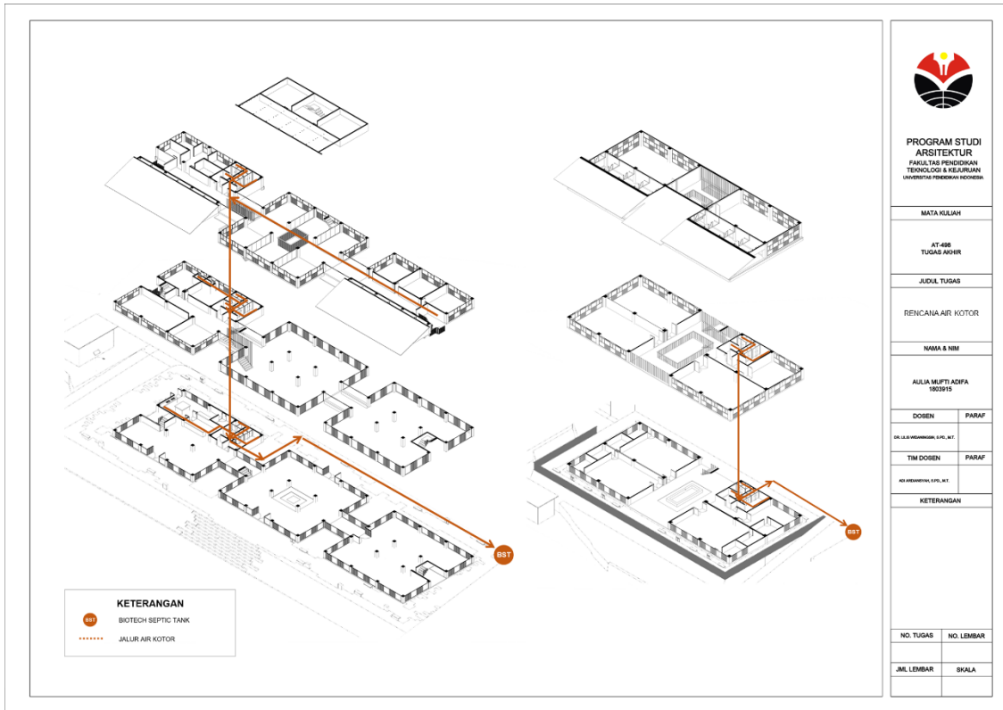
Gambar 5.18 Rencana Air Kotor
