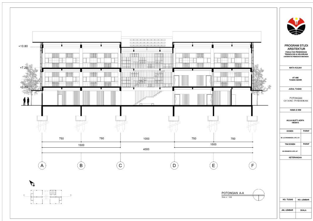
Gambar 5.14 Potongan Gedung Pendidikan
