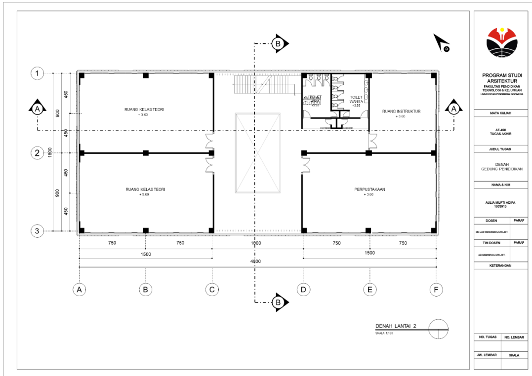
Gambar 5.5 Denah Gedung Pendidikan Lantai 2
