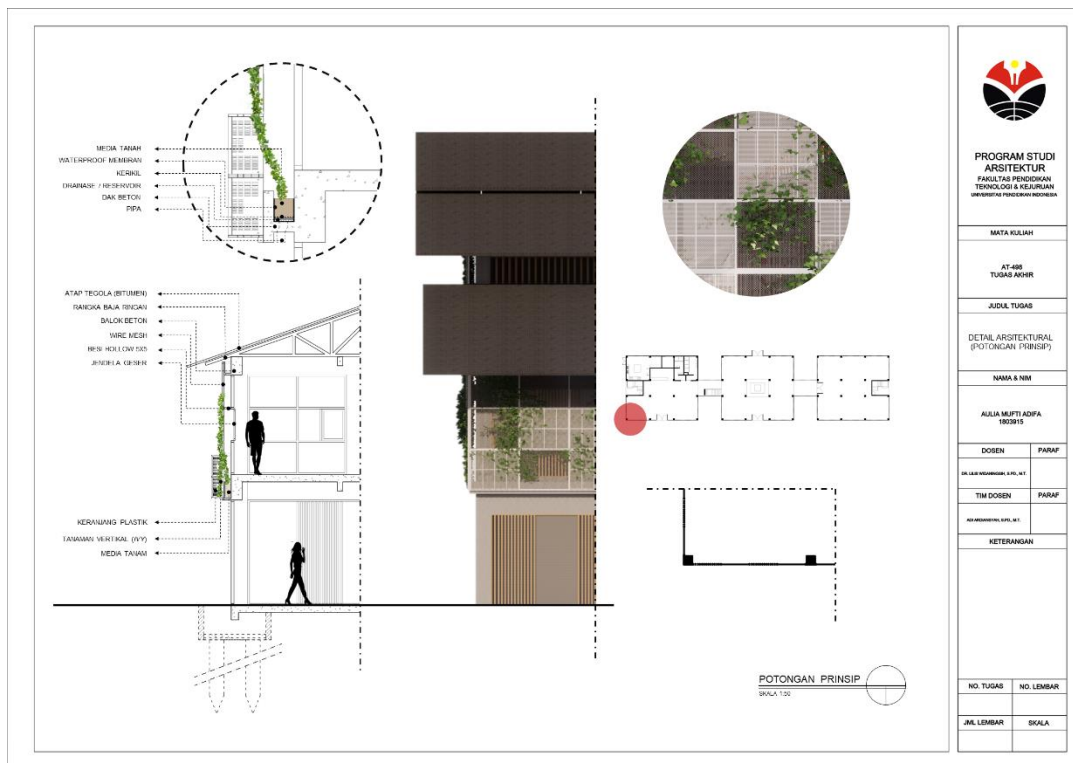
Gambar 5.22 Potongan Prinsip
