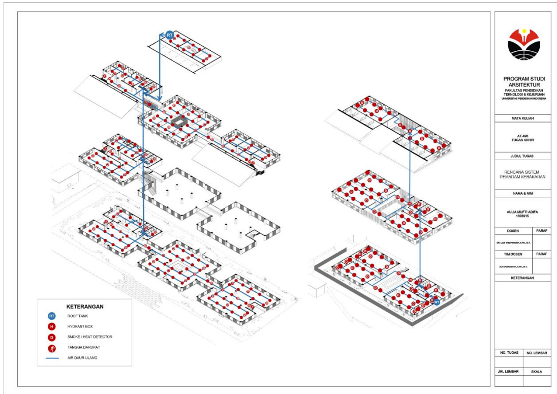
Gambar 5.20 Rencana Sistem Pemadam Kebakaran Sumber: Penulis, 2022
