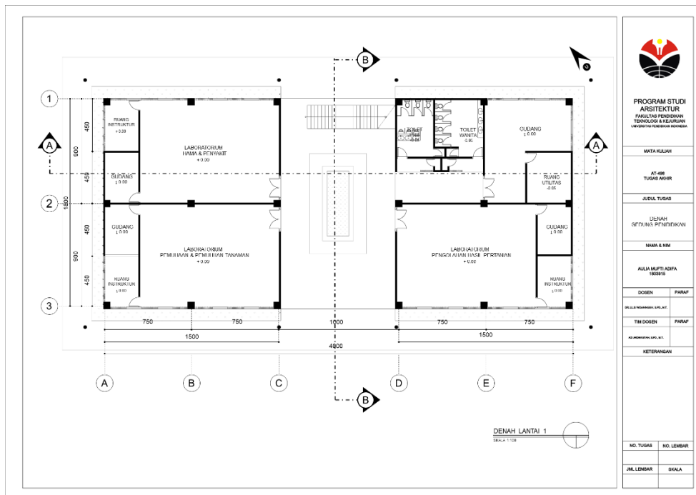
Gambar 5.4 Denah Gedung Pendidikan Lantai 1 Sumber: Penulis, 2022
