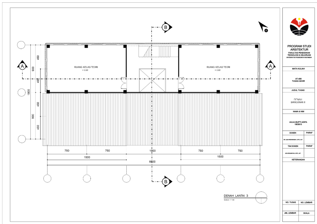
Gambar 5.6 Denah Gedung Pendidikan Lantai 3
