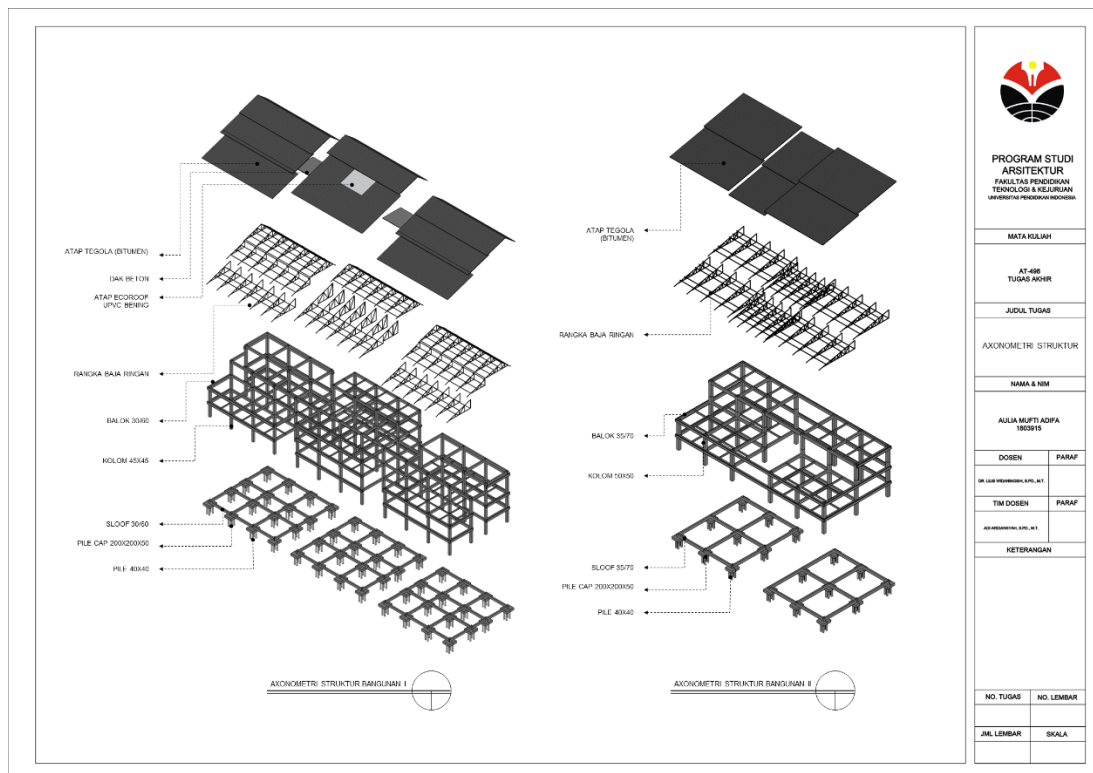
Gambar 5.16 Axonometri Struktur Bangunan
