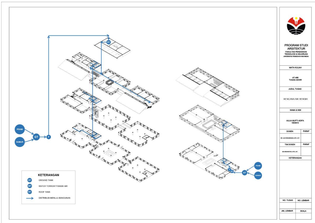
Gambar 5.17 Rencana Air Bersih Sumber: Penulis, 2022
