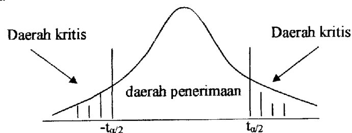
Gambar 3.1 Uji Dua Arah atau Two-Tail Test
