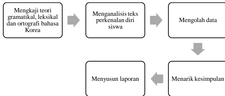
Gambar 3.1 Desain Penelitian
