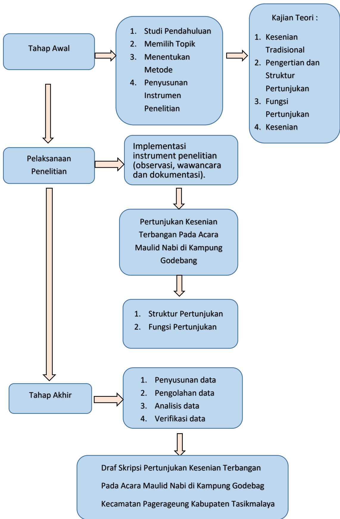
Gambar 3.1. Desain Penelitian
