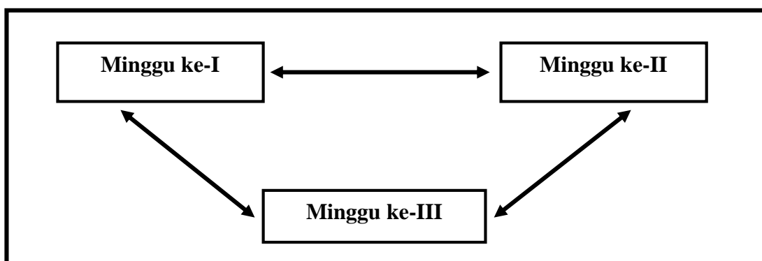
Gambar 3.3 Triangulasi Waktu
