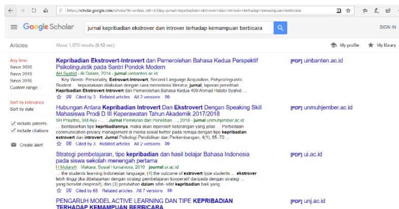
Gambar 3.4 Hasil Pencarian
