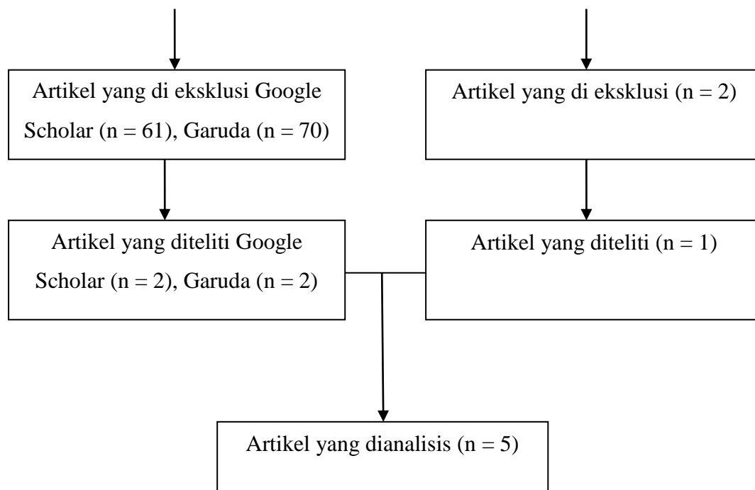
Gambar 3. 1 Bagan PRISMA
