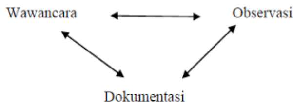
Gambar 3.2 Teknik Triangulasi
