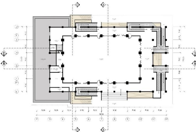
Gambar 5. 3 Denah lantai 1 (redesain) Masjid Besar Lembang (Sumber: Dokumentasi penulis, 2018)
