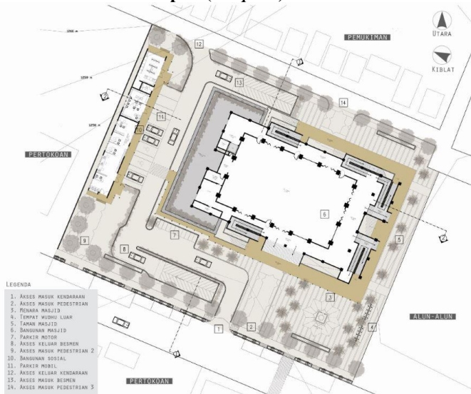
Gambar 5.1 Rencana tapak (redesain) Masjid Besar Lembang (Sumber: Dokumentasi penulis, 2018)
