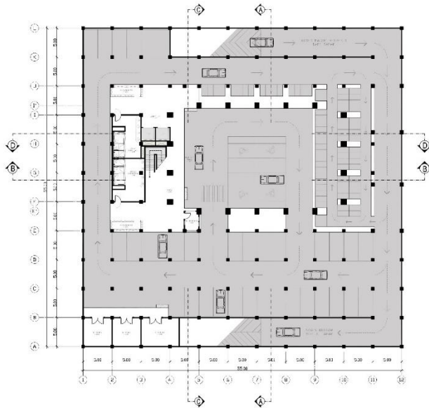
Gambar 5. 6 Denah lantai besmen 1 Masjid Besar Lembang (Sumber: Dokumentasi penulis, 2018)
