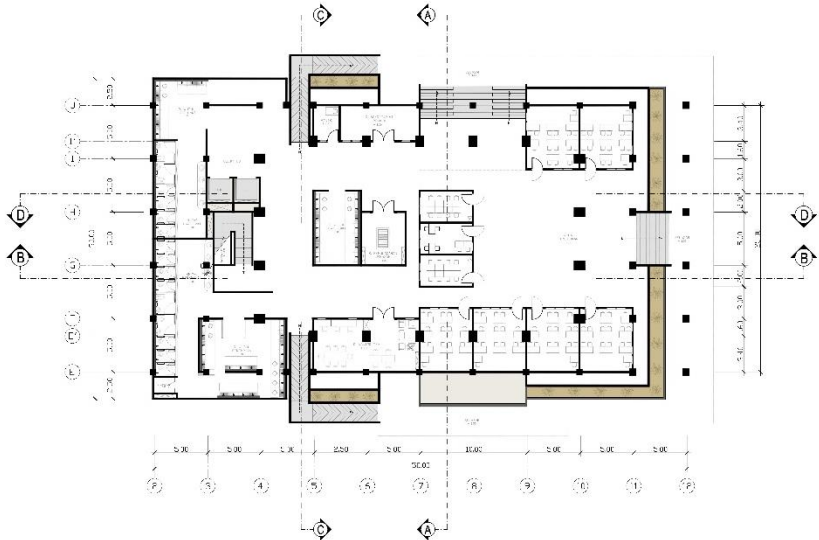
Gambar 5. 4 Denah lantai semibesmen Masjid Besar Lembang (Sumber: Dokumentasi penulis, 2018)
