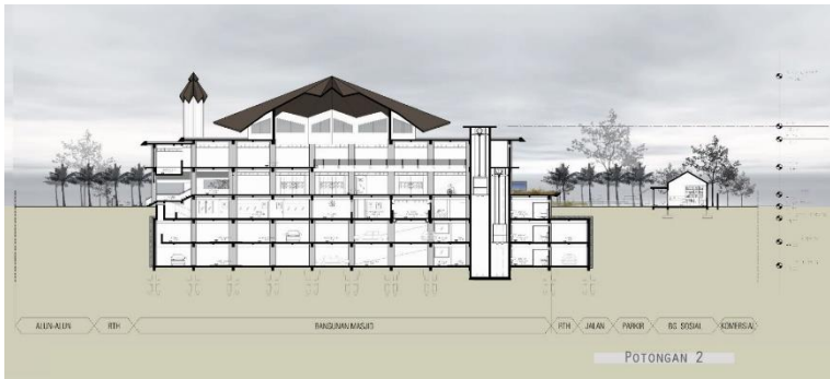
Gambar 5. 12 Potongan 2 Masjid Besar Lembang (Sumber: Dokumentasi penulis, 2018)
