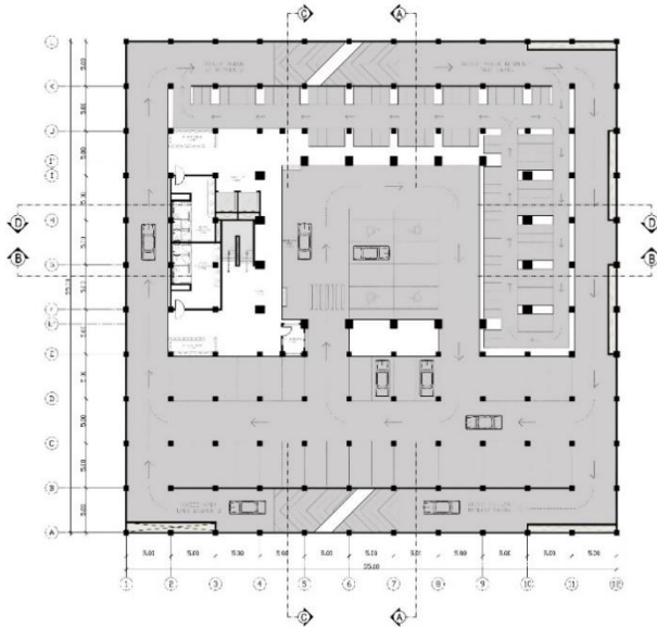
Gambar 5. 5 Denah lantai besmen 2 Masjid Besar Lembang (Sumber: Dokumentasi penulis, 2018)
