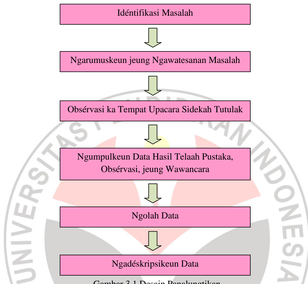
Gambar 3.1 Desain Panalungtikan
