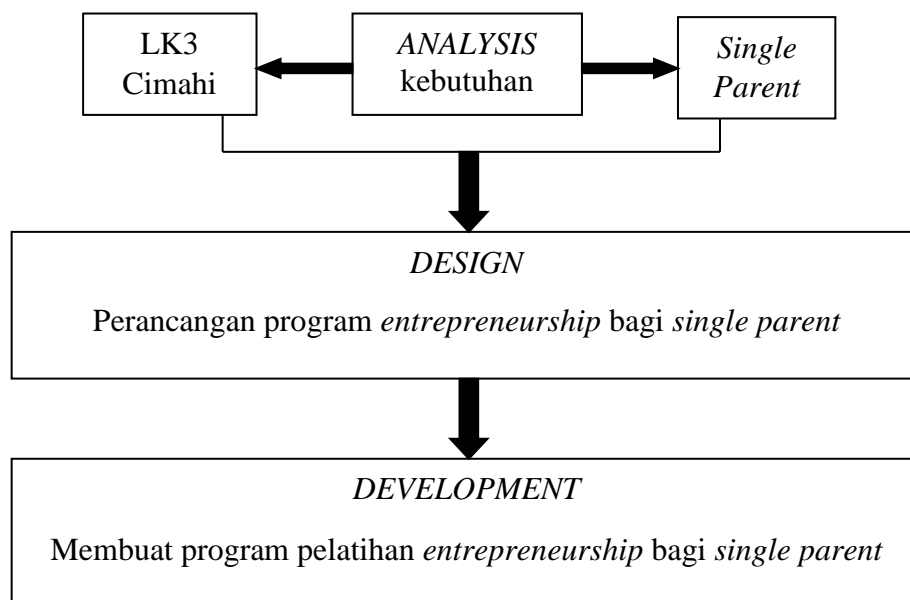
Gambar 3.1 Desain Penelitian
