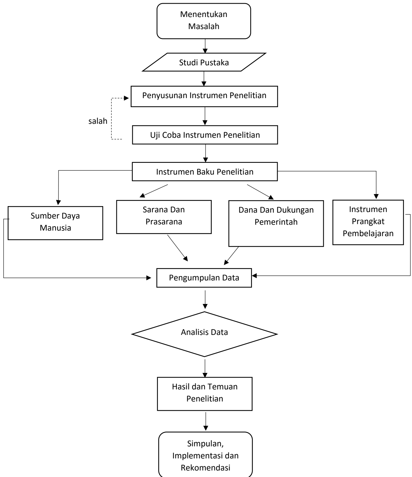
Gambar 3.1 Langkah-Langkah Penelitian
