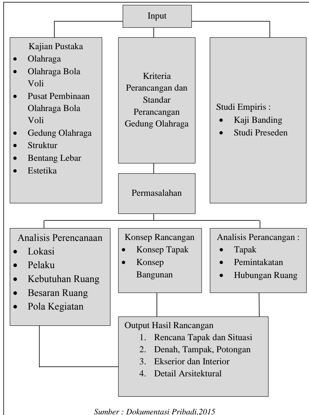
Diagram 1.1 Kerangka Berpikir
