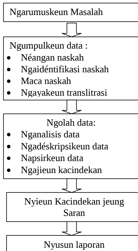
Gambar 3.1 Desain Panalungtikan
