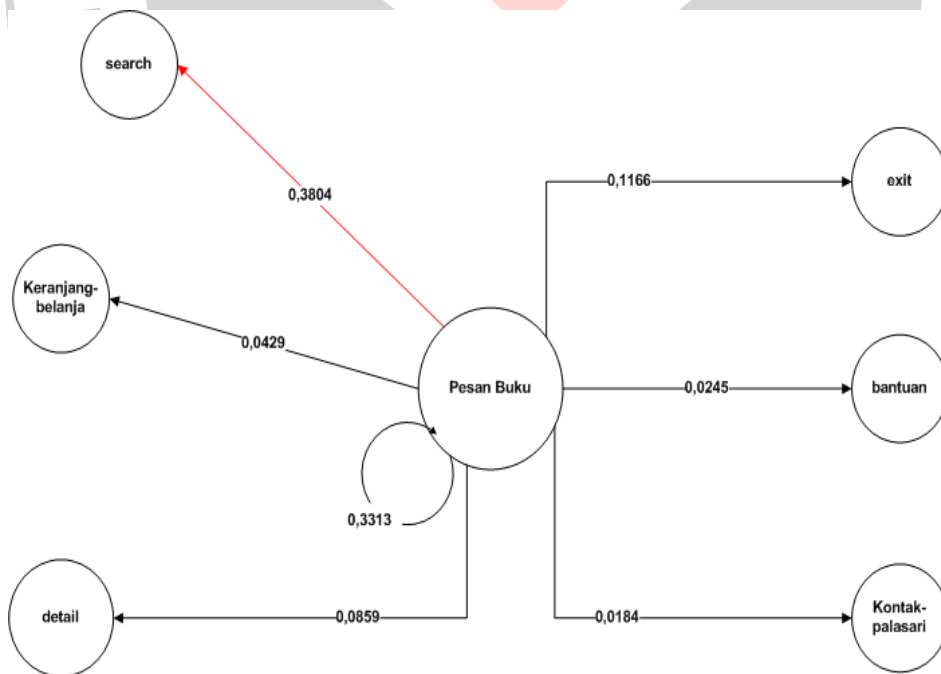
CBMG Fungsi Daftar Buku Best Seller
