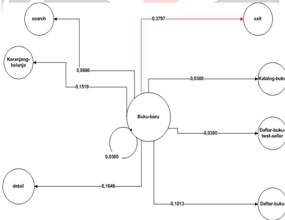
CBMG Fungsi Konfirmasi Pembayaran
