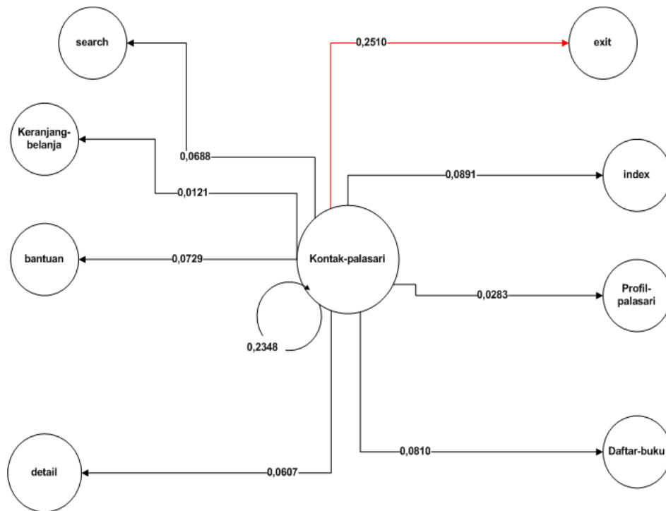
CBMG Fungsi Kontak Palasari
