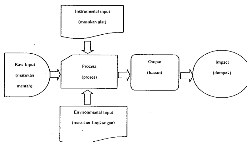
Gambar 2 Pendekatan Sistem
