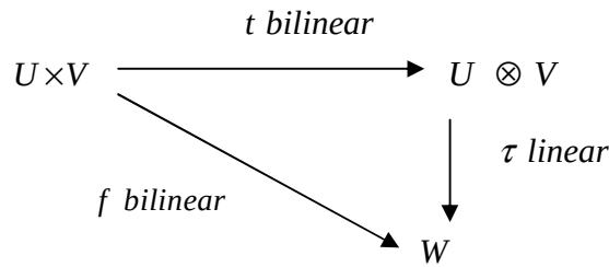
Gambar 3.1 Sifat Universal Hasilkali Tensor
