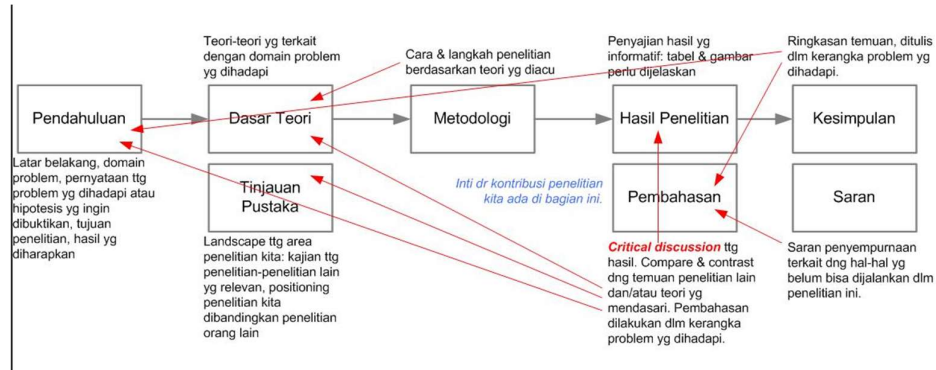
Gambar 1.1 Struktur Tesis
